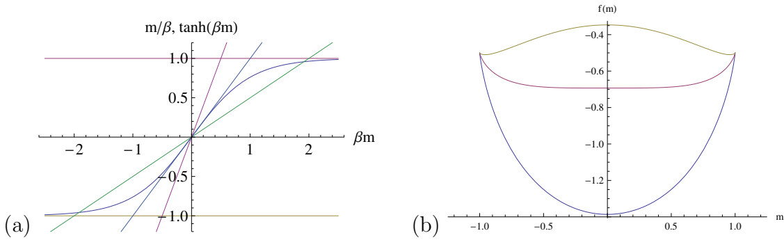
図 4.6: (a) 自己無撞着方程式 (4.56) のグラフによる解法 (図 4.5 と同じ) . 直線は, パラメタの値は, zJ = 1, \beta = 0.5, 1, 2 . (b) 平均場近似 (ブラッグ-ウィリアムズ近似) での磁化の関数としての自由エネルギー f(T, m) . 自由エネルギーの値は (a) の交点に相当する極大, 極小の点は図 4.5 と同じである .
