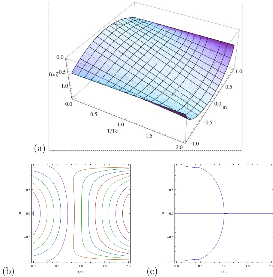
図 4.7: (a) 温度と磁化の関数としての自由エネルギー f(T, m) . (b) 自由エネルギー f(T, m) の等エネルギー曲線 . (c) 自由エネルギー f(T, m) の極値を表す ( ) 式の解曲線 . m = \pm 1 付近でがたついているのは計算精度が悪いため、なめらかに m = \pm 1 に近づいていく .
