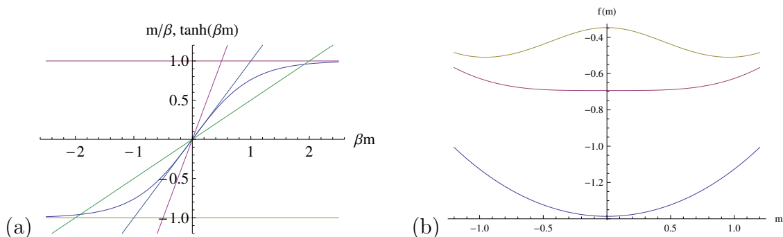
図 4.5: (a) 自己無撞着方程式 (4.56) のグラフによる解法．直線は，パラメタの値は， zJ = 1 ， \beta = 0.5, 1, 2 ．(b) Ising モデルの平均場近似での計算に現れる f(T, m) の形．自由エネルギーの値は (a) の交点に相当する，極大，極小の点でのみ意味を持つ．
